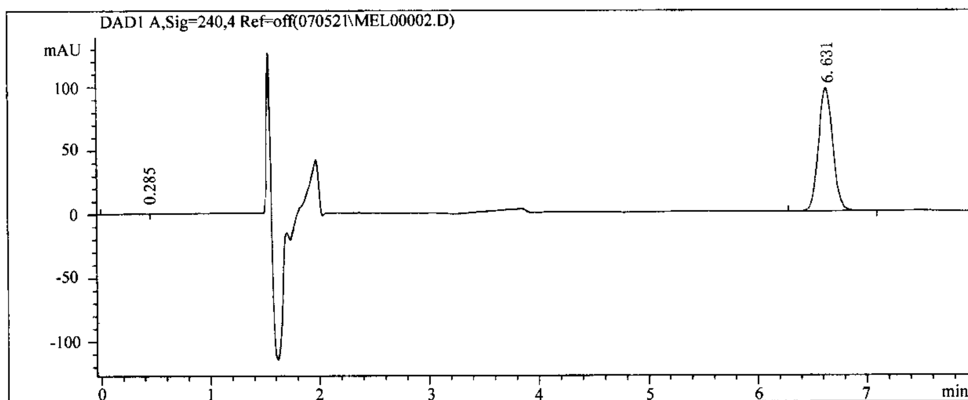
图 A.1 三聚氰胺标准色谱图
