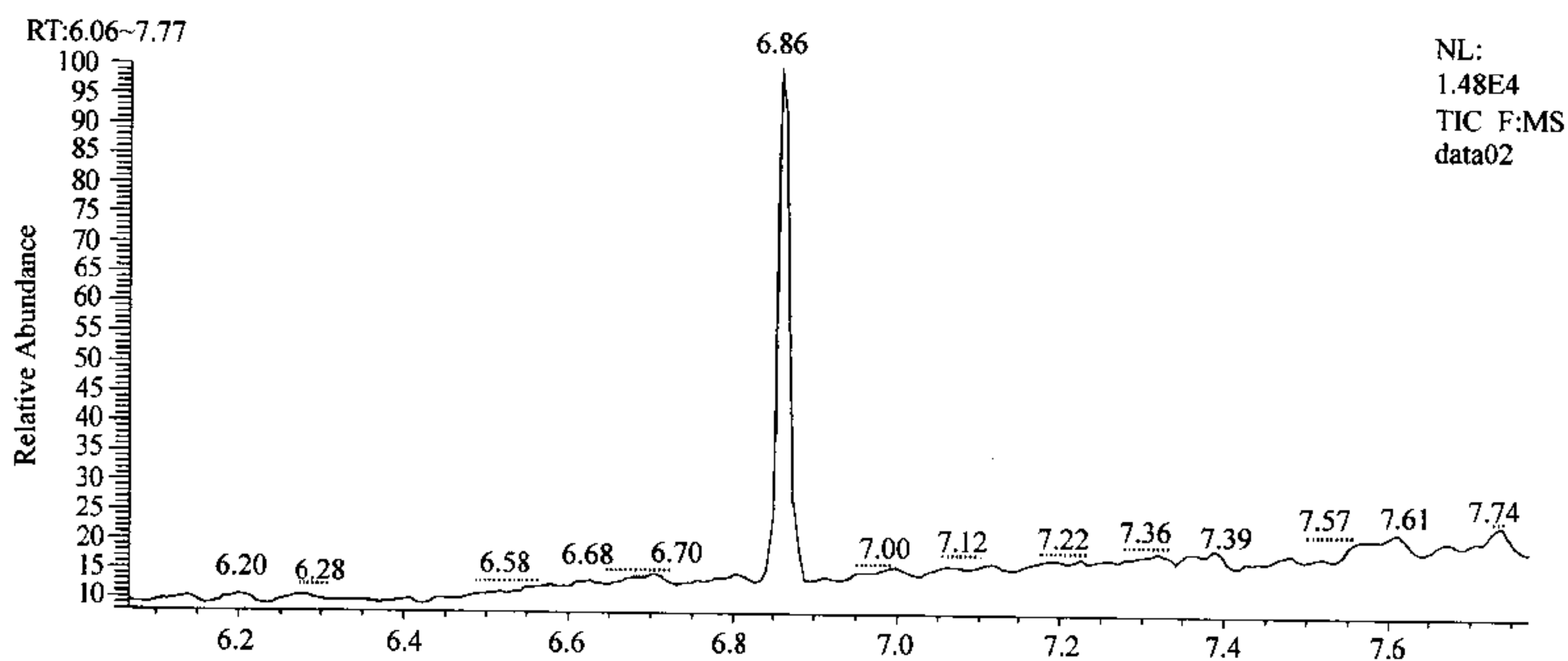
图 A.3 三聚氰胺标准品衍生物选择离子色谱图
