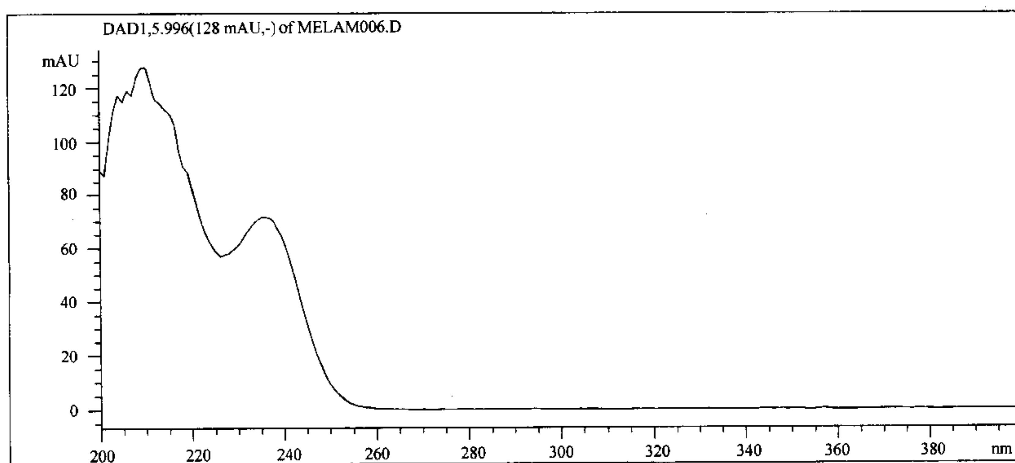
图 A.2 三聚氰胺紫外光谱图
